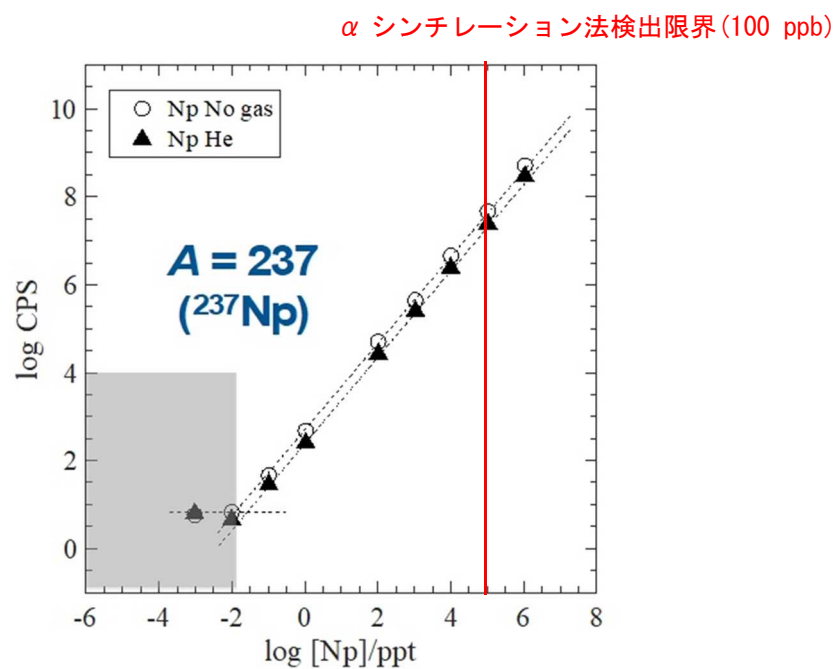
図8 ICP-MS で測定した ^{237}\text{Np} の検量線
